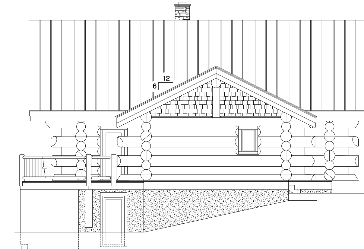
Right Elevation
