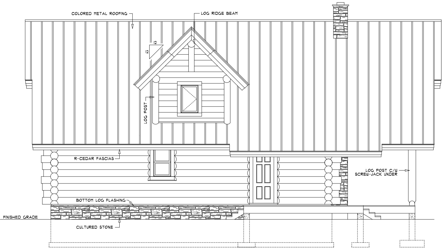
Right Elevation
